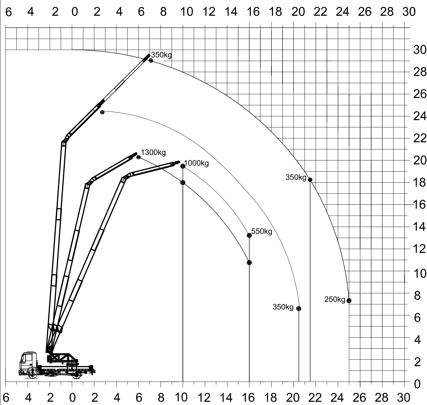
Belastungsdiagramm K25-30TS
