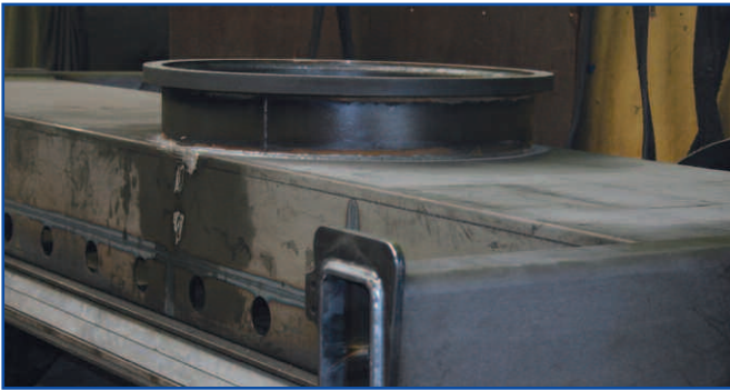
Komplett geschlossene Stahlwanne bedeutet wenig Torsion
