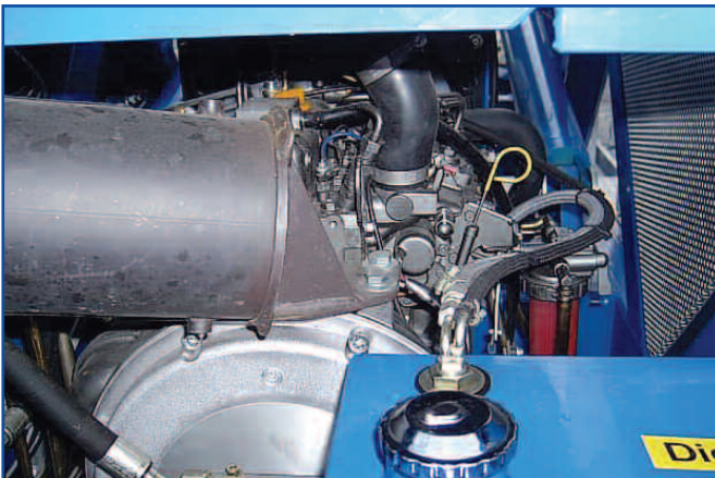
Dieselmotor serienmäßig
