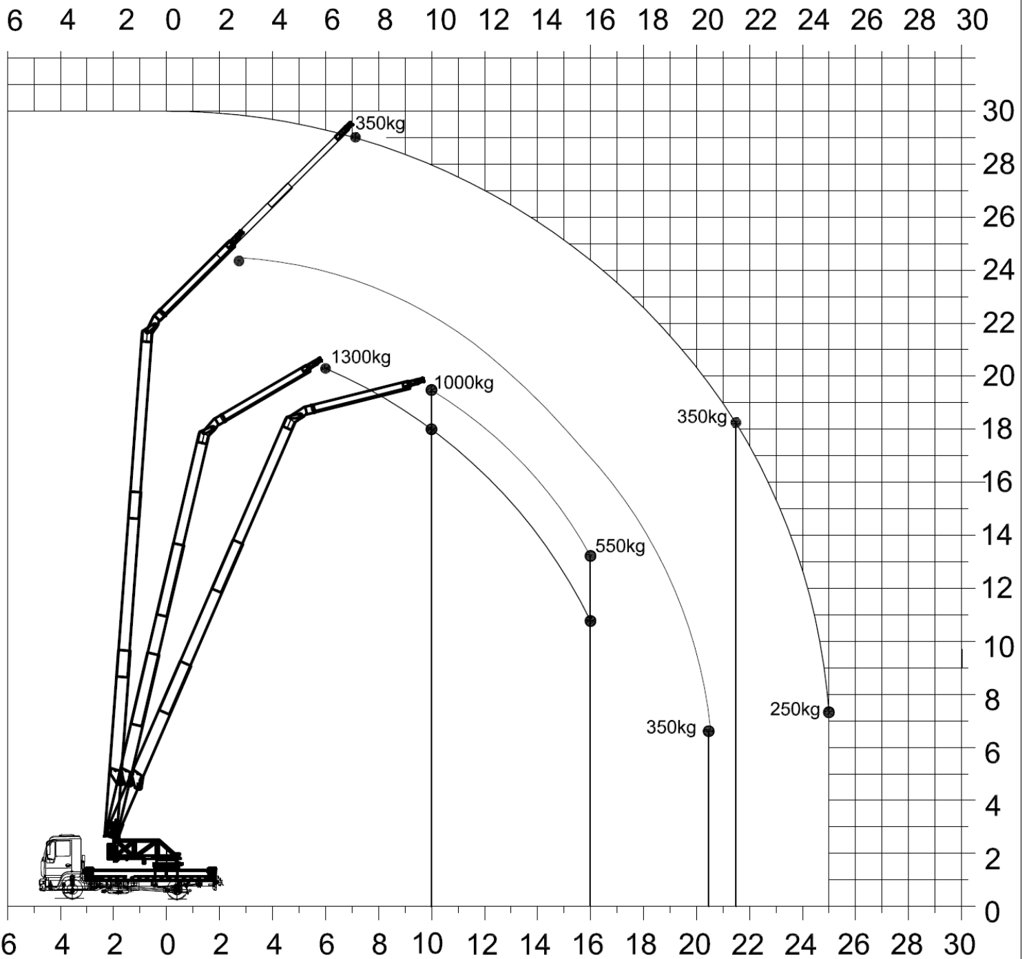
Belastungsdiagramm K25-30TS
